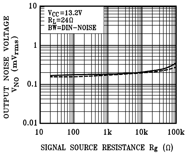
V_{NO} - R_g
