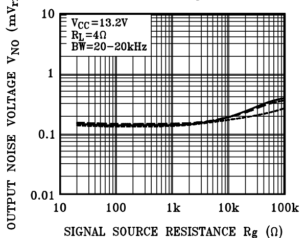
V_{NO} - R_g
